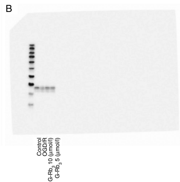
Fig.2A: Bcl-2
